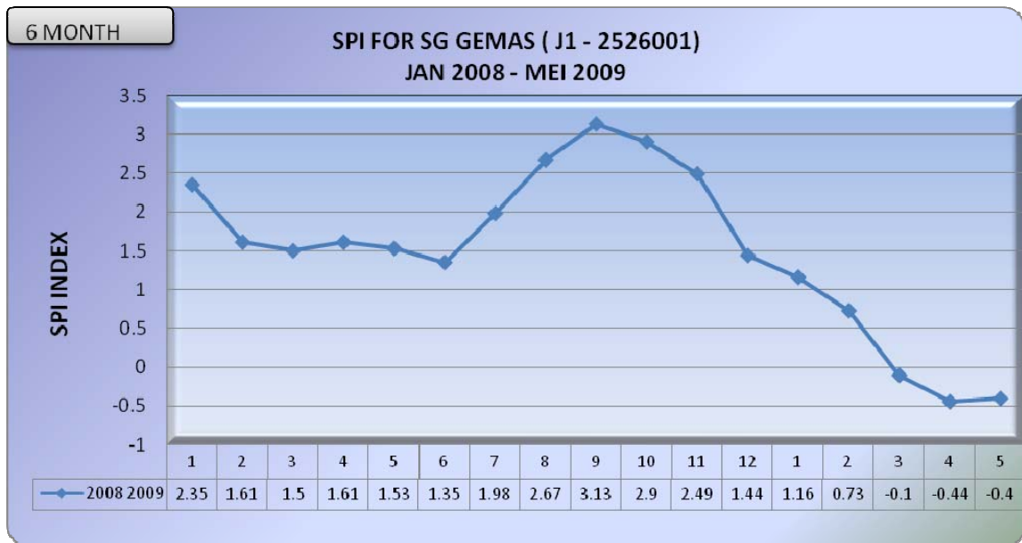
Rajah 11 : Graf SPI untuk Stesen Ladang Sungai Gemas (J1) (6 bulan)
