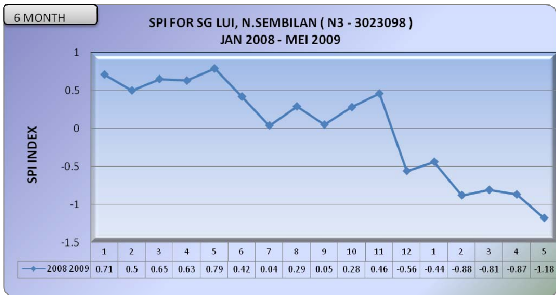
Rajah 7 : Graf SPI untuk Sungai Lui Halt (N3) (6 bulan)
