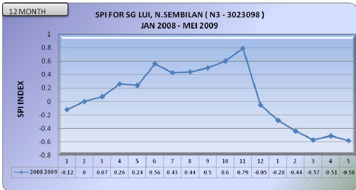
Rajah 8 : Graf SPI untuk Sungai Lui Halt (N3) (12 bulan)
