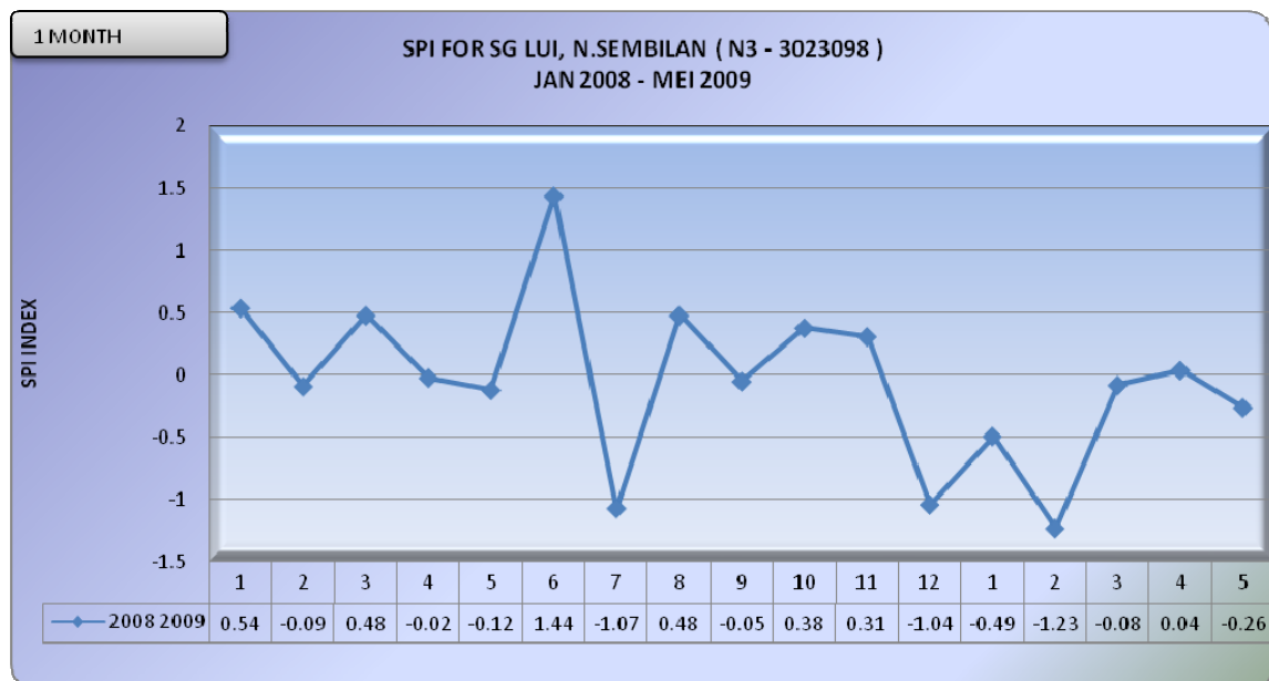
Rajah 5: Graf SPI untuk Sungai Lui Halt (N3) (1 bulan)
