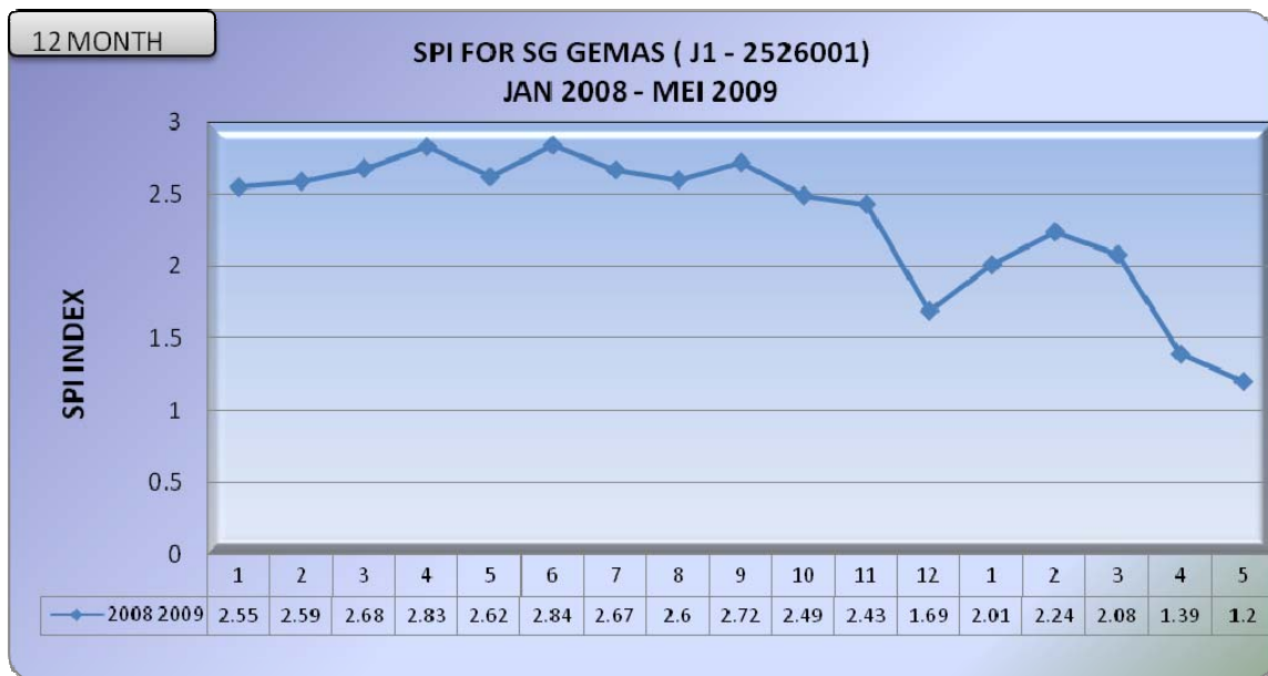
Rajah 12 : Graf SPI untuk Stesen Ladang Sungai Gemas (J1) (12 bulan)
