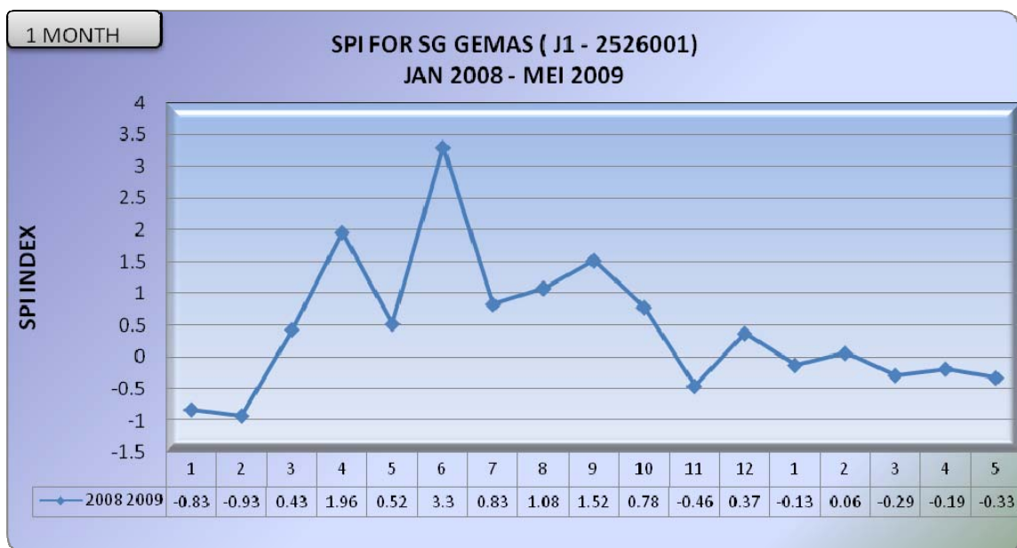
Rajah 9 : Graf SPI untuk Stesen Ladang Sungai Gemas (J1) (1 bulan)
