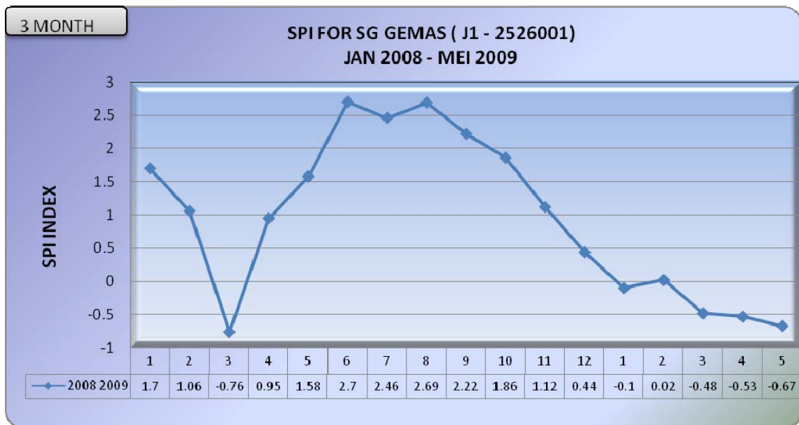
Rajah 10 : Graf SPI untuk Stesen Ladang Sungai Gemas (J1) (3 bulan)
