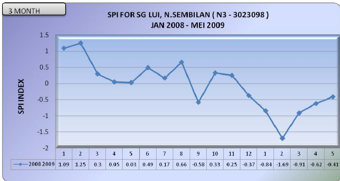
Rajah 6 : Graf SPI untuk Sungai Lui Halt (N3) (3 bulan)
